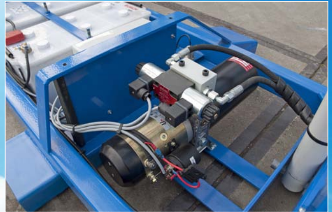
Elektro-hydraulisch
